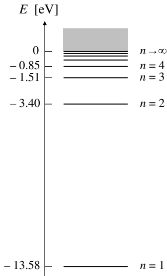
Obr. 5a. Energie stacionárních stavů atomu vodíku.
