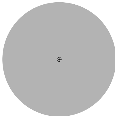
Obr. 1. Jaderný (Rutherfordův) model atomu.
