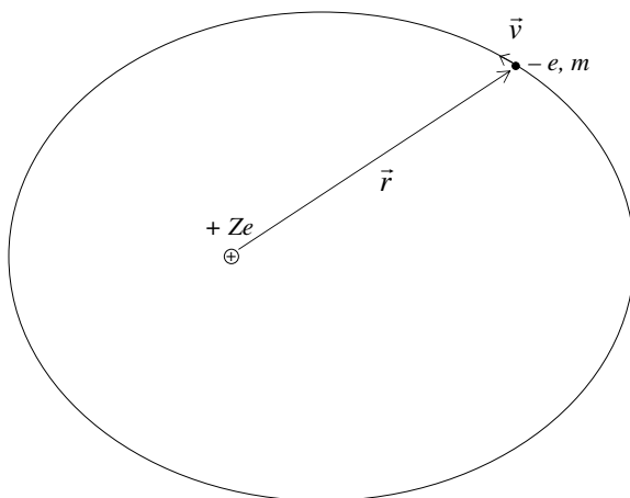
Obr. 2. Planetární model atomu.
