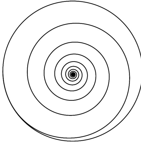
Obr. 4. Kolaps planetárního atomu.
