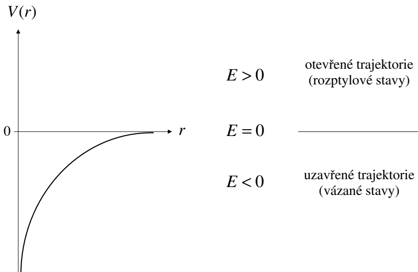
Obr. 3. Závislost charakteru řešení Keplerova problému na hodnotě energie.
