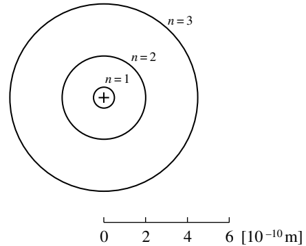
Obr. 5b. Kruhové dráhy elektronu v Bohrově modelu atomu vodíku.
