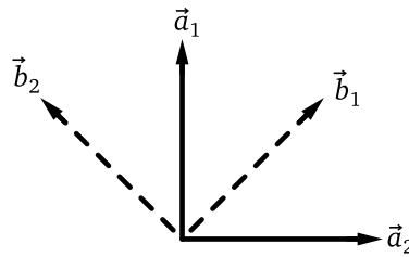
Obr. 3. Jedna z možností voľby Blochových vektorov pre merania A_1, A_2, B_1 a B_2 , ktoré vedú k maximálnemu narušeniu CHSH nerovnosti (4). Konkrétne si môžeme vziať horizontálny smer ako smer x a vertikálny ako smer z
