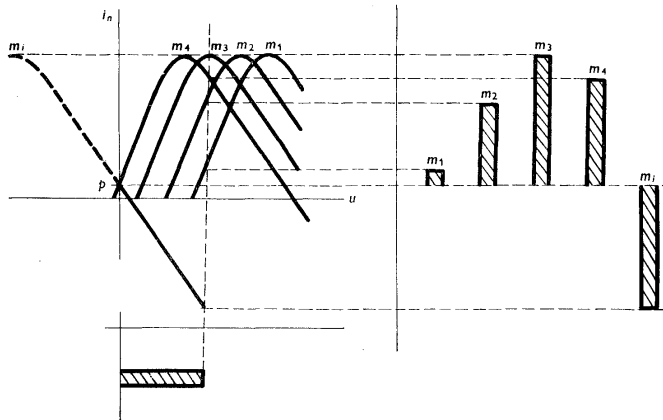
Obr. 3. Přenosové charakteristiky vstupního dílu i = f(u) pro různé stavy paměti m_1 až m_4 (excitační stavy) a m_1 (inhibiční stav). Naznačen je přenos vstupního signálu u na výstup i_m , jak se uplatňuje na vstupu a-\zeta převodníku s prahem p .
