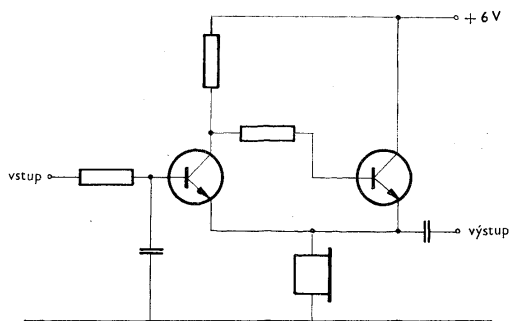
Obr. 5. Schéma převodníku pro přeměnu analogového signálu ve formě stejnosměrného proudu na kmitočty výstupních impulsů konstantní amplitudy.
