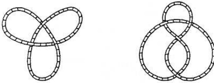
Obr. 1. Schematické znázornění dvou zauzlených křivek.
