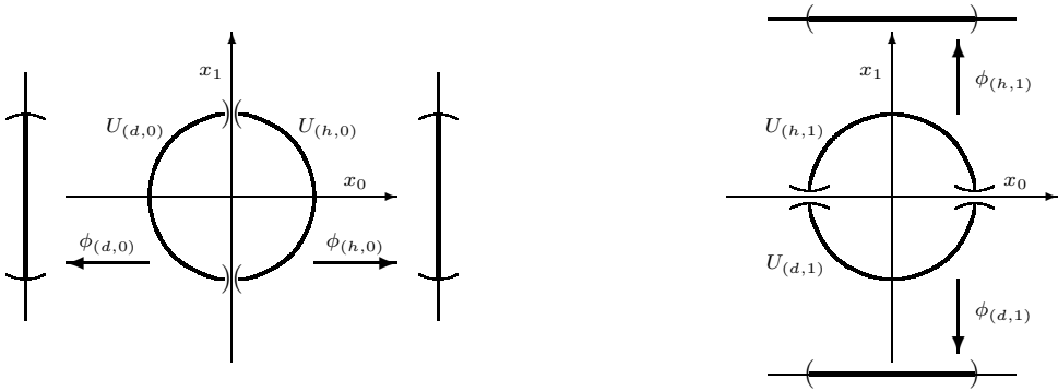
Obr. 2. Atlas \mathcal{A}_0 pokrývá kružnici S^1 čtyřmi otevřenými polokružnicemi. Mapující zobrazení jsou homeomorfiny na otevřené podintervaly \mathbb{R}^1 .
