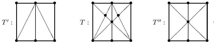
Obr. 3. Tři triangulace čtverce.
