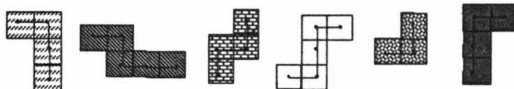
Obrázek 9: Grafové kódování
