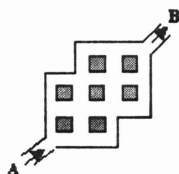
Obrázek 2: Bludiště
