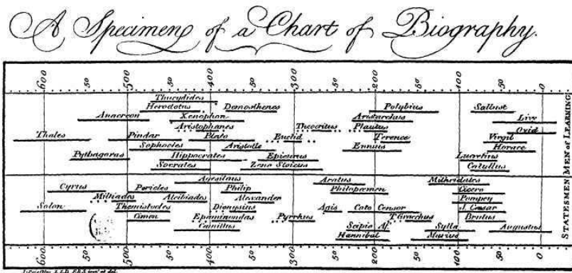
Obr. 20: Druhá čtvrtina diagramu J. Priestleye (1765).
