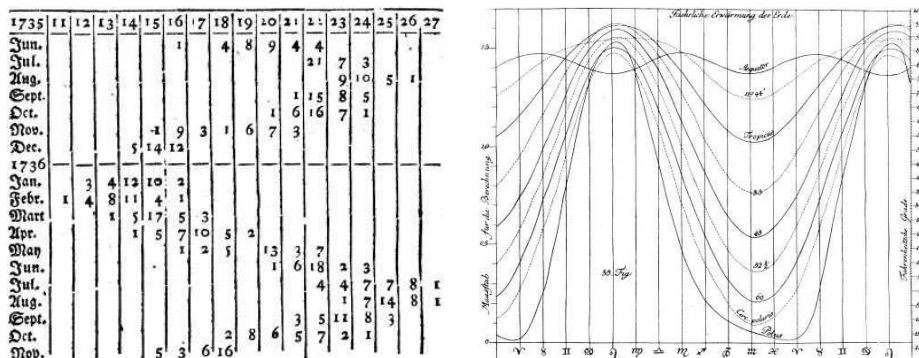
Obr. 22: Lambertův „číselný graf“ (1779) udávající počet dnů v měsíci, kdy bylo dosaženo určité teploty (horizontální osa ve ^{\circ}\text{C} ) a graf závislosti ohřevu půdy v průběhu roku na zeměpisné šířce.
