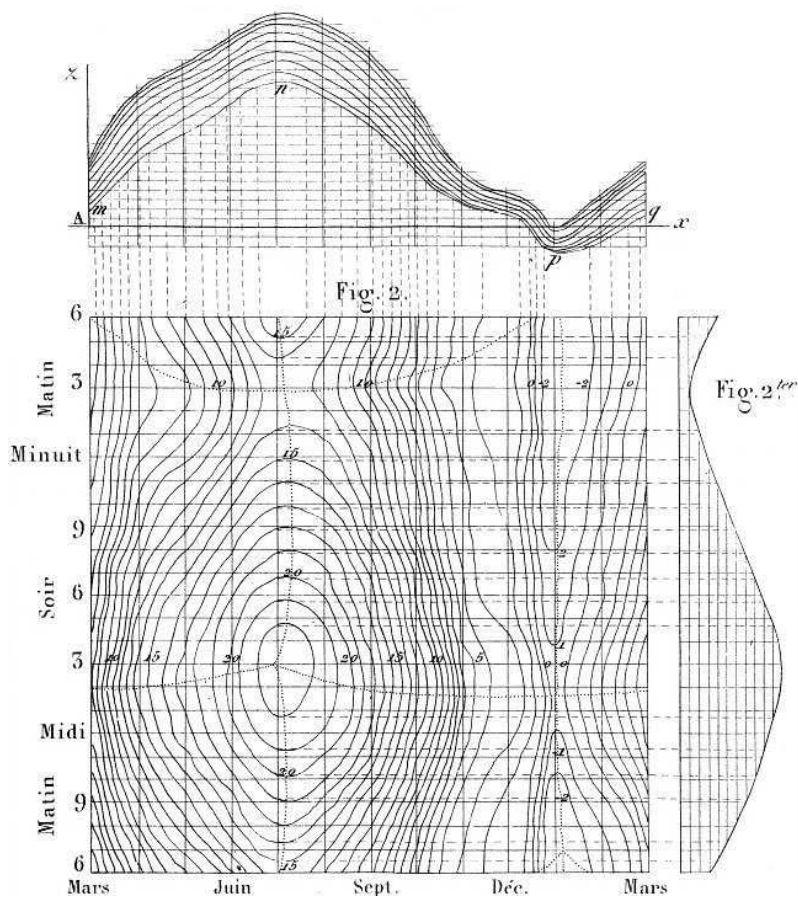
Obr. 29: Lalanneův prostorový graf {měsíce \times hodiny \times teplota} (1845).
